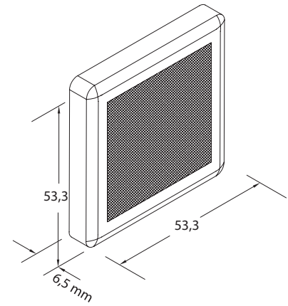
Wymiary oprawy / Fixture dimensions / Размеры светильника
