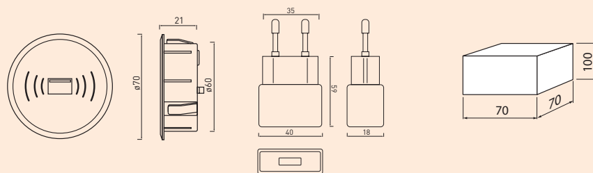
Wymiary ładowarki, wymiary zasilacza
