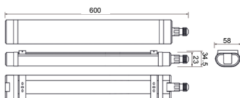
LD-HOU18W06-NB
