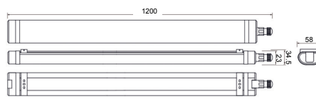
LD-HOU36W12-NB
