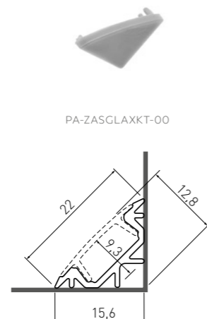
Zaślepka / End cap / Заглушка / кінцевий ковпачок:
